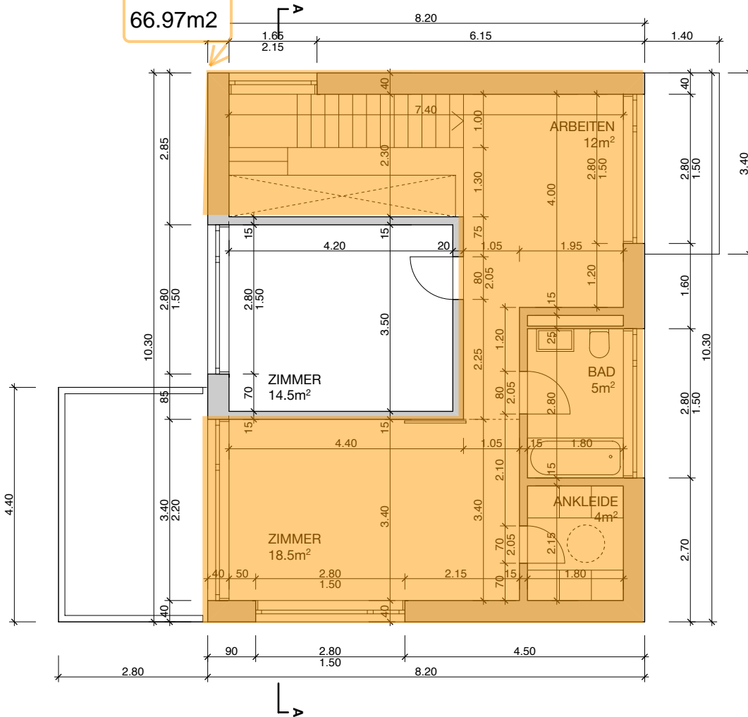
OBERGESCHOSS 1:100
