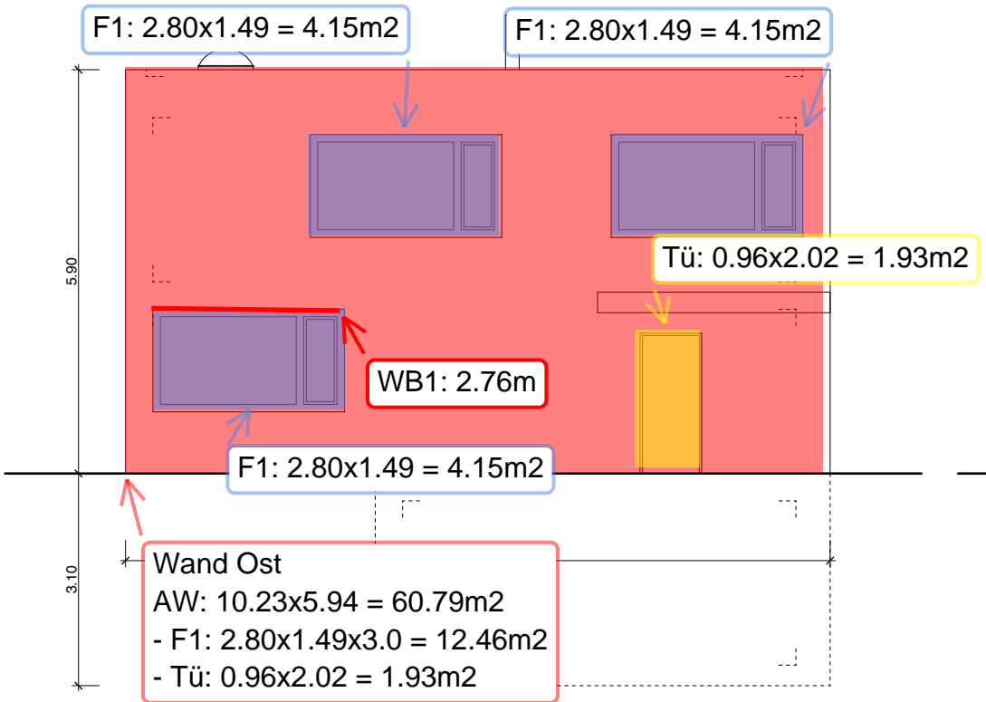
ANSICHT OST 1:100
